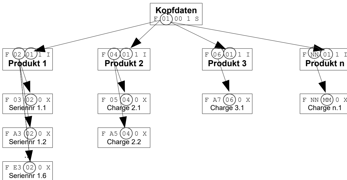
Abbildung 7: Graphische Darstellung der Ebenen
