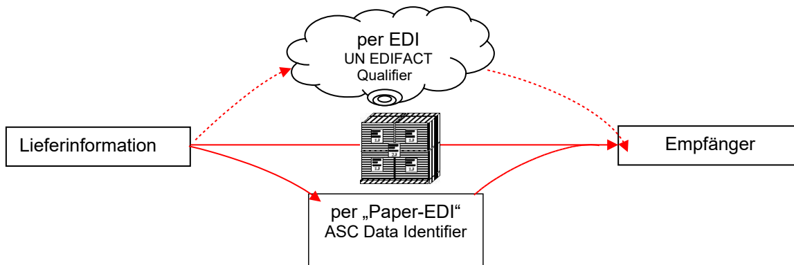
Abbildung 5: Skizze Kompatibilität der Syntax „UN EDIFACT - Qualifier“ und „ISO/IEC 15418 – ASC Data Identifier“
