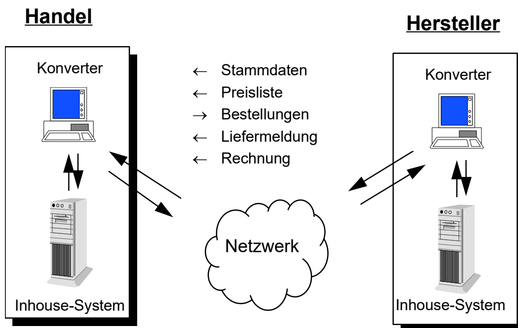
Abbildung 1: Komponenten der EDI-Anwendung
